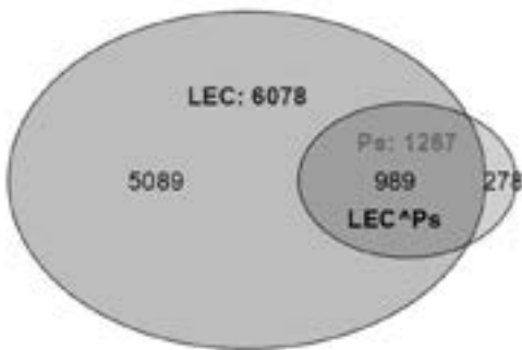
Fig. 4. LEC y Poesía cósmica. NLE = 278 ; PLE = 278 / 1267 = 0.219
