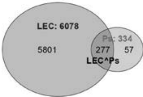
Fig. 3. LEC y Poesía cósmica en comparación. Verbo.
