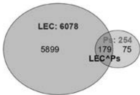
Fig. 1. LEC y Poesía cósmica en comparación. Adjetivo.
