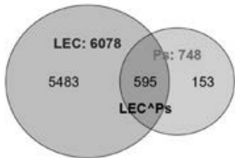
Fig. 2. LEC y Poesía cósmica en comparación. Nombre.
