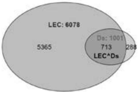
Fig. 6. LEC y Don Quijote de la Mancha NLE = 288 ; PLE = 288 / 1001 = 0.288
