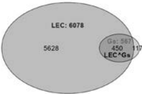
Fig. 5. LEC y Génesis del Antiguo testamento. NLE = 117 ; PLE = 117 / 567 = 0.206
